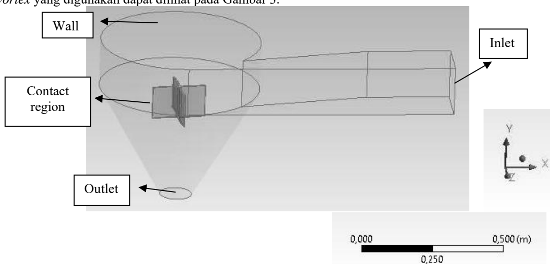
Gambar 3. Pemodelan Komputasi dan Penetapan Kondisi Batas Pada Turbin Reaksi Vortex Ultra-Low Head .
