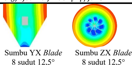
Gambar 10. Kontur Distribusi Pressure Pada Turbin Dengan Variasi Jumlah Dan Sudut Blade .
