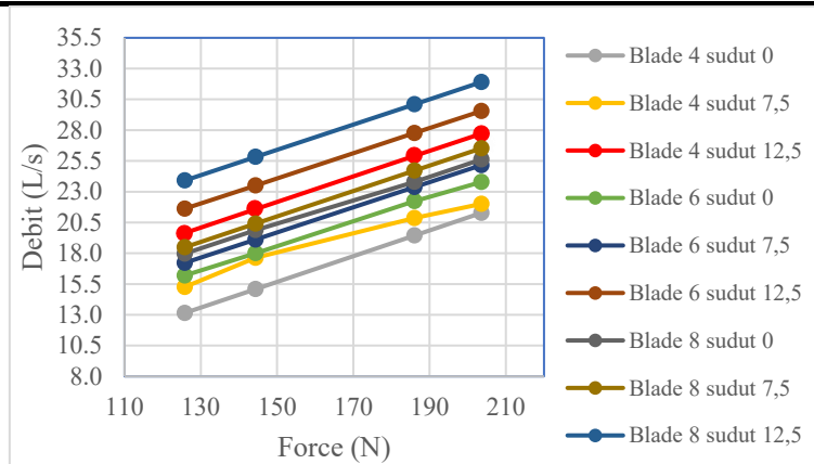
Gambar 9. Nilai Force Terhadap Debit
