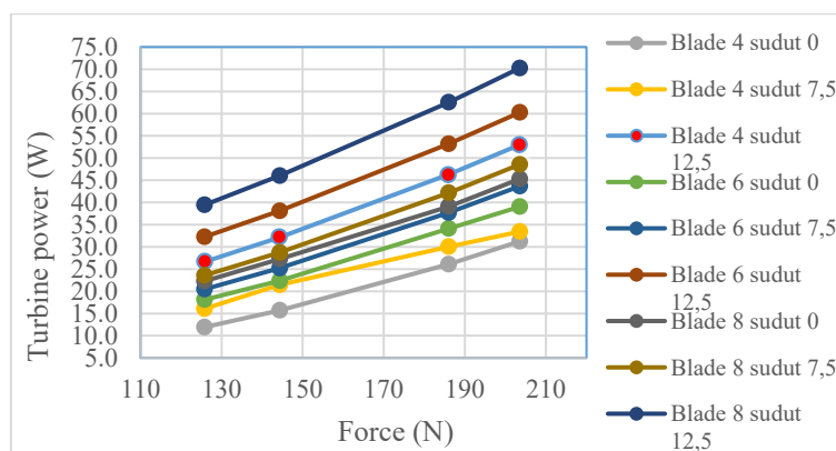
Gambar 11. Nilai Force Terhadap Daya.
