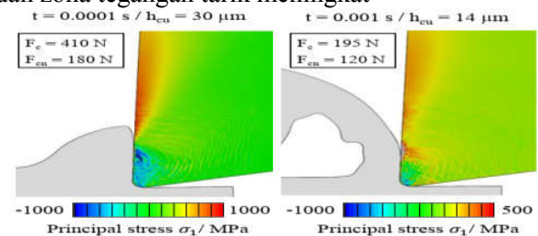
Gambar 3 Gambaran Umum Distribusi Tegangan Utama \sigma_1 untuk alat dengan r\beta = 10 \mu\text{m} setelah t_c = 0.1 \text{ ms} (masuknya alat pemotong) dan kemudian t_c = 1 \text{ ms} .
