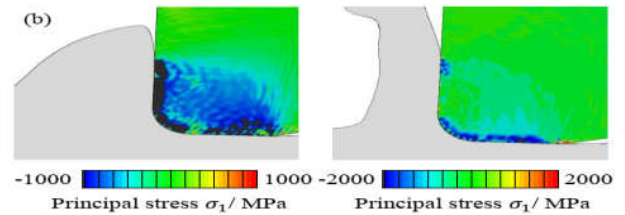
Gambar 5. Distribusi tegangan utama \sigma_1 untuk alat dengan r_{\beta} = 20 \mu\text{m} dan VB = 60 \mu\text{m} tanpa (a) dan dengan (b) tegangan sisa
