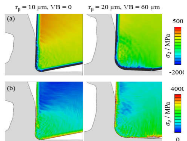
Gambar 6. Distribusi (a) tegangan utama \sigma_2 dan dari (b) tegangan setara von Mises \sigma_v untuk t = 0.001 s.
