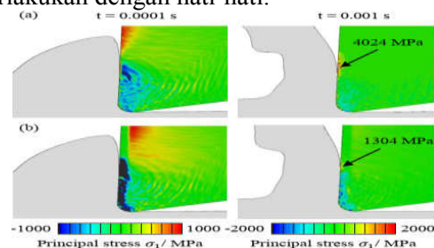
Gambar 4. Analisis rinci tegangan utama \sigma_1 untuk alat referensi tanpa (a) dan dengan (b) tegangan sisa.
